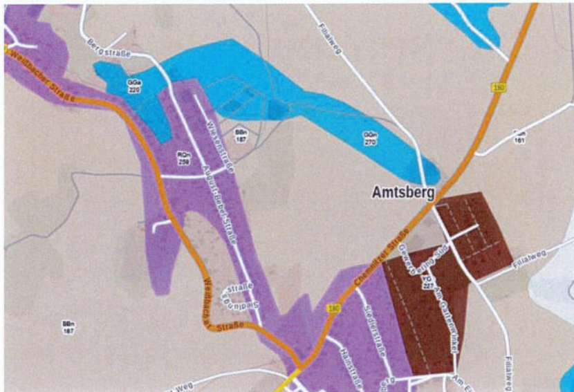
Abbildung 9: Bodenkarte 1:50.000, iDA - interdisziplinäre Daten und Auswertungen, LfULG
