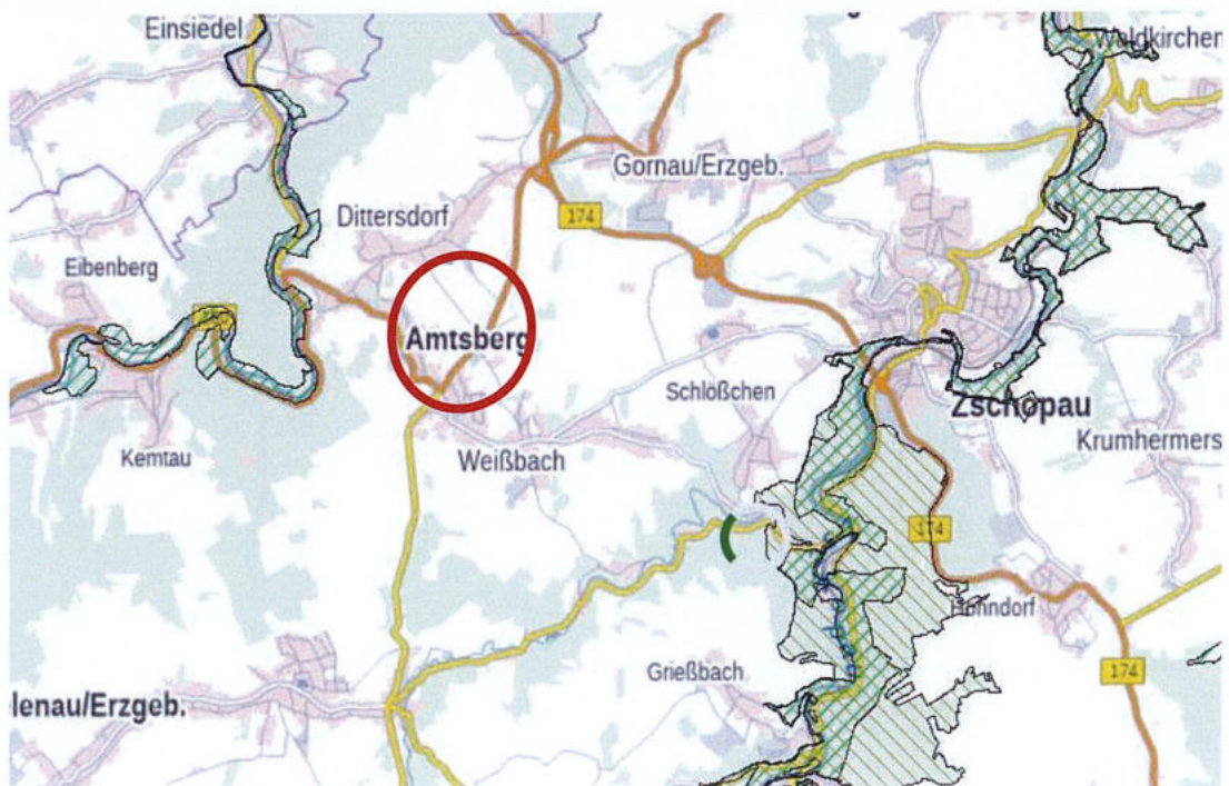
Abbildung 10: FFH-Gebiete im Umfeld des Planungsgebietes ( iDA – interdisziplinäre Daten und Auswertungen, LfULG)
